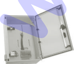
06CTEL-A-PT Caixa telecontagem tipo A para PT
